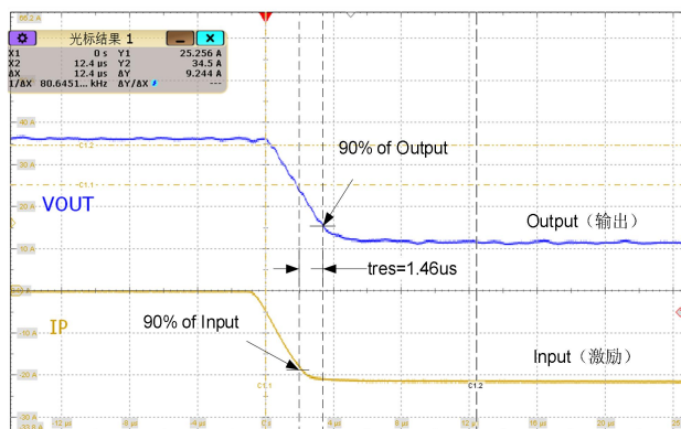
传输响应负向下降波形
