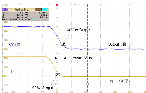
传输响应正向下降波形
