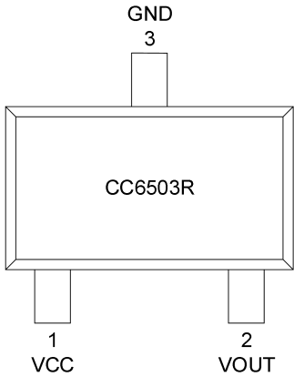
SOT23-3 封装
