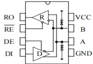
图 1 引脚分布图
