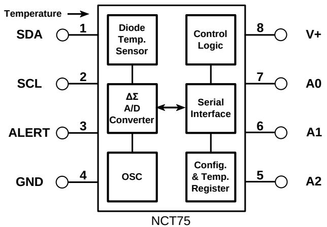
图 1 NCT75内部各模块示意图
