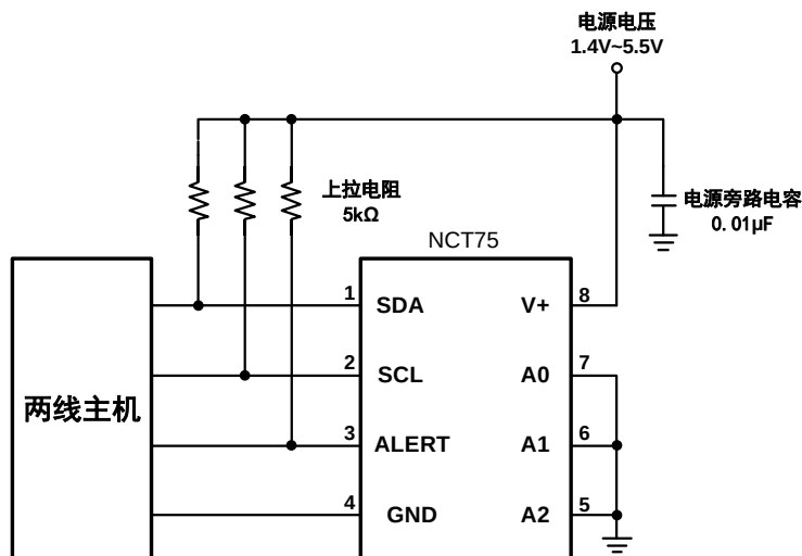
图 7 NCT75的典型连接方式
