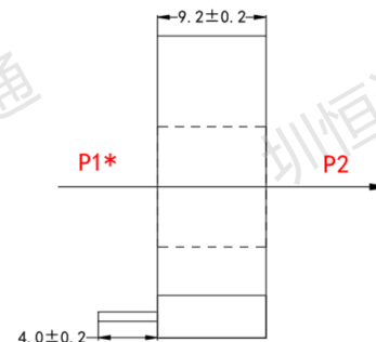
侧视图
