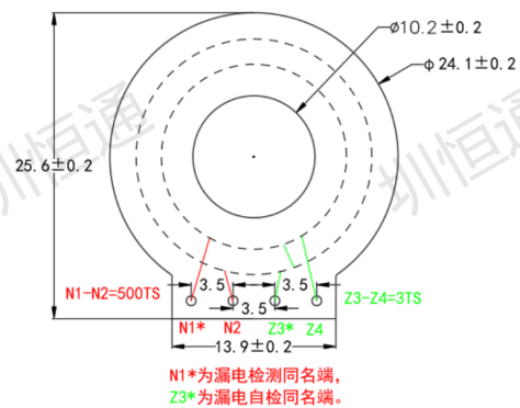
主视图
