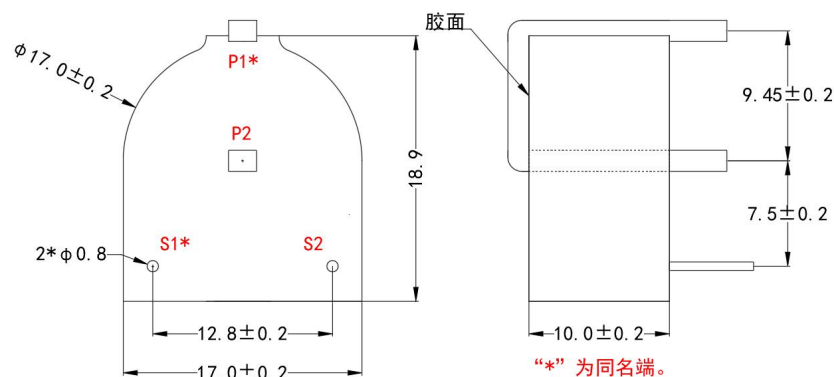
主视图
