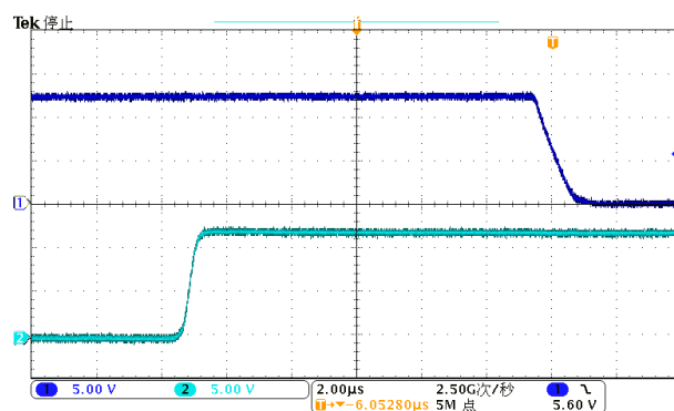
t_{\text{DEAD}}@V_{\text{DD}}=12\text{V}
