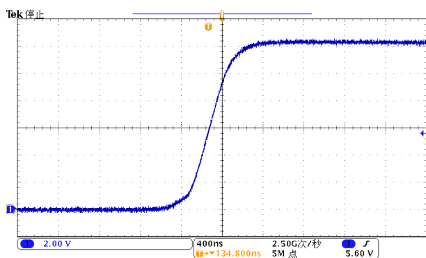
t_r @ V_{DD}=12V
