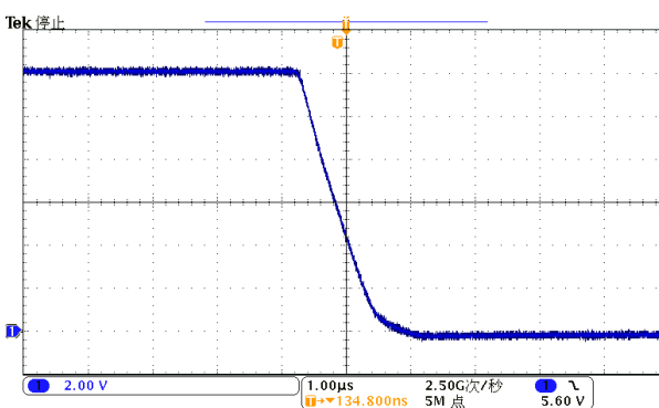
t_f @ V_{DD}=12V
