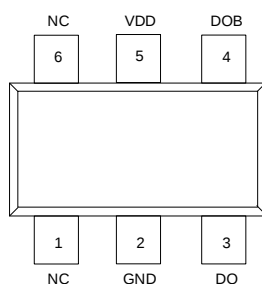
TSOT23-6L
