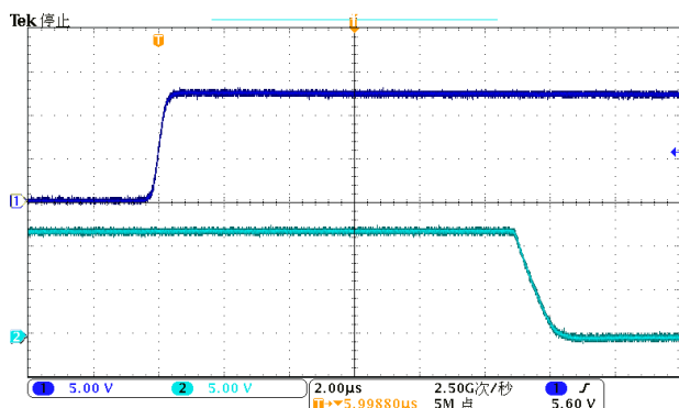
t_{\text{DEAD}}@V_{\text{DD}}=12\text{V}
