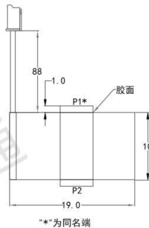
底视图
