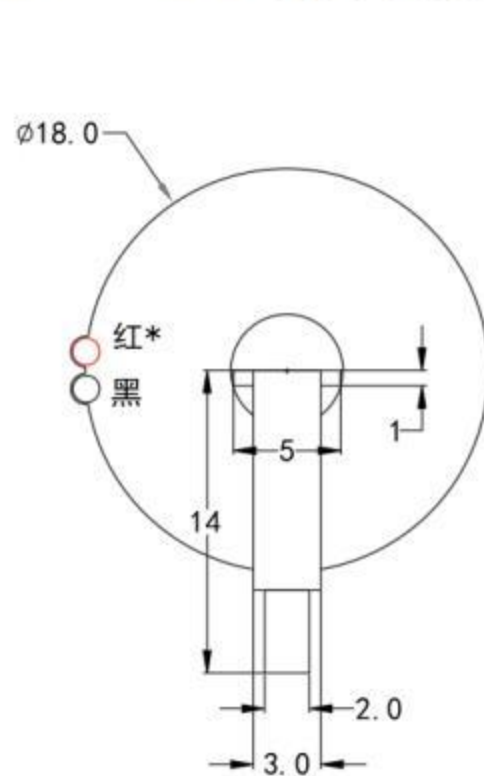
主视图
