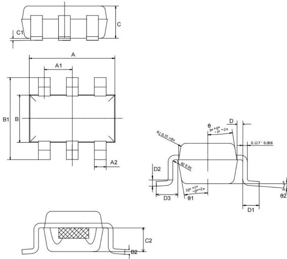
SOT23-6L 12/14排框架
