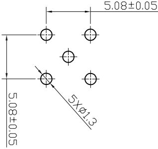
建议PCB印刷尺寸
