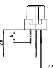
Solder lug
