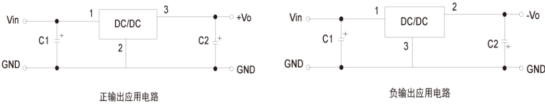
图 2 典型应用电路
