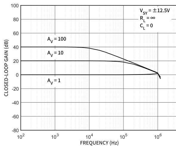
图 18 闭环增益与频率的关系 ( \pm 12.5V )
