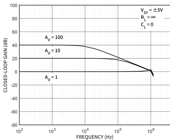
图 17 闭环增益与频率的关系 ( \pm 5V )
