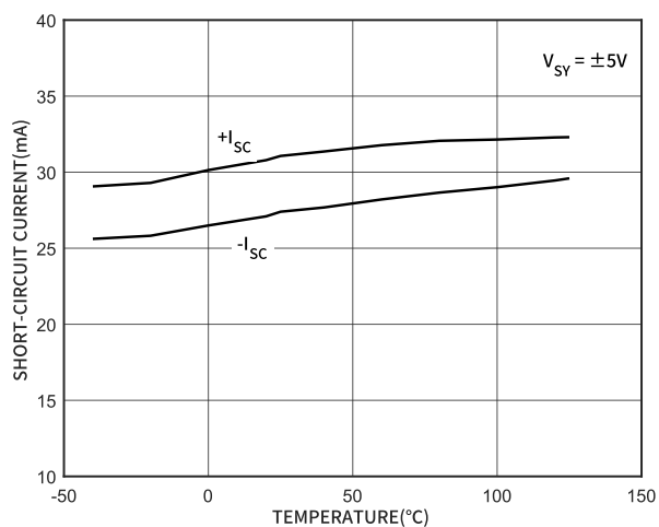
图 5 短路电流的温度特性 ( \pm 5V )
