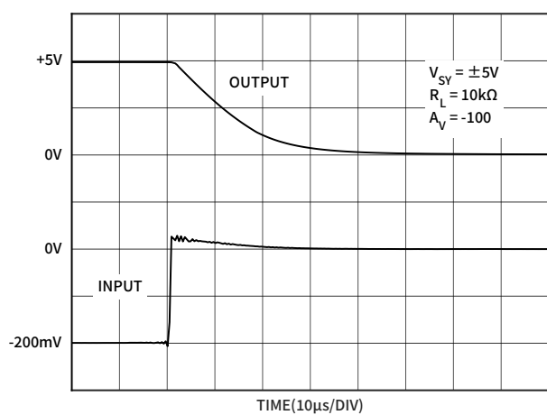
图 15 负过压恢复时间 ( \pm 5V )
