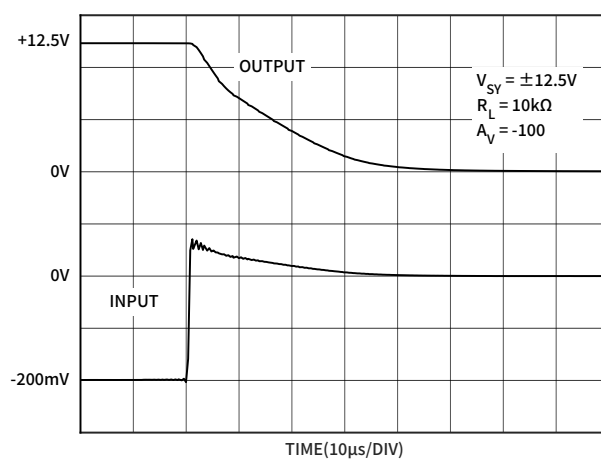
图 16 负过压恢复时间 ( \pm 12.5V )
