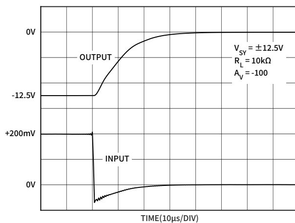
图 14 正过压恢复时间 ( \pm 12.5V )
