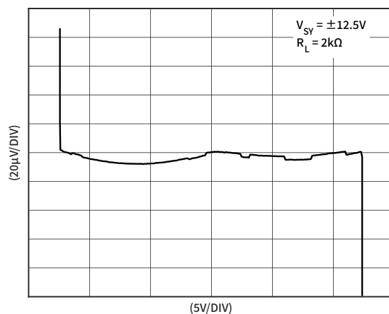
图 31 增益线性度
