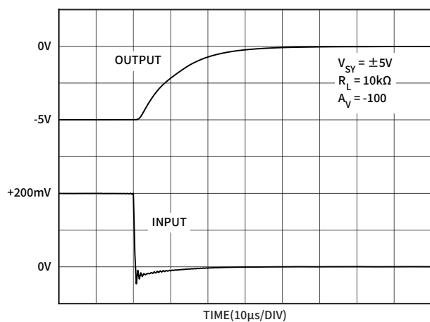
图 13 正过压恢复时间 ( \pm 5V )
