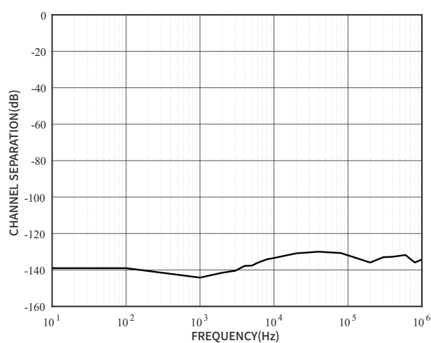
图 28 通道隔离度
