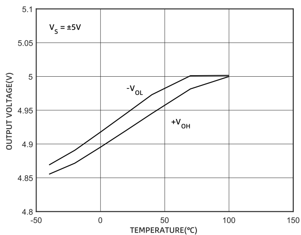
图 5 输出电压摆幅的温度特性 (±5V)
