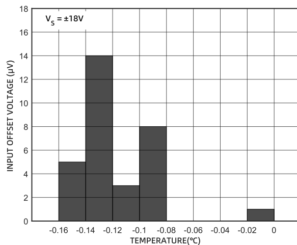
图 4 输入失调电压漂移分布图 (±18V)
