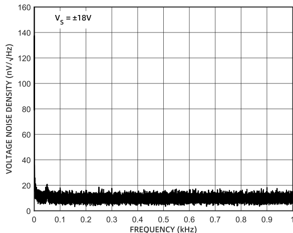
图 26 噪声频谱密度图 (±18V)
