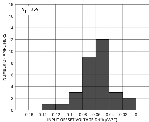
图 3 输入失调电压漂移分布图 (±5V)
