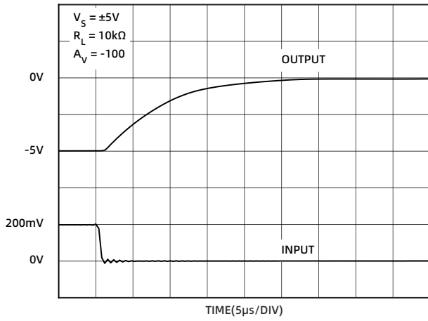
图 19 正过载恢复时间 (±5V)
