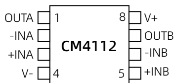
MSOP8
