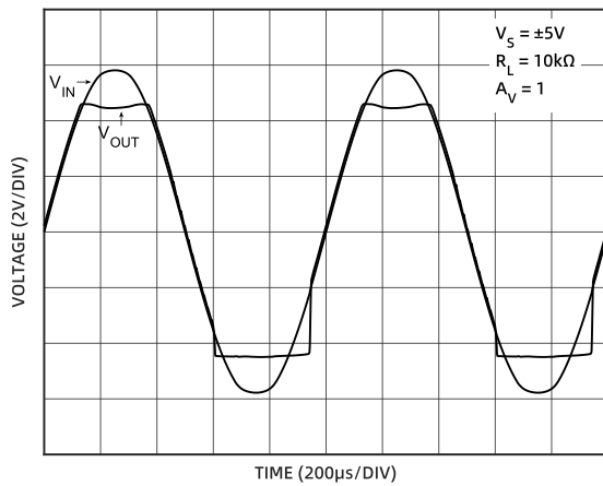
图 27 无反相 (±5V)
