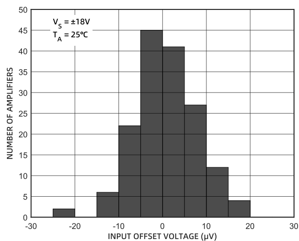
图 2 输入失调电压分布图 (±18V)
