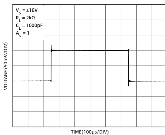
图 16 小信号瞬态响应 (±18V)
