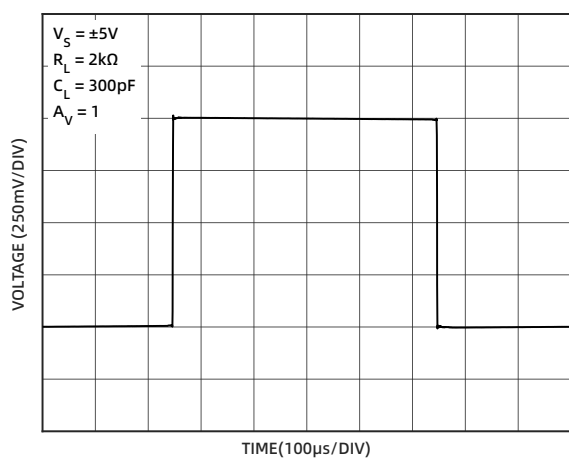
图 17 大信号瞬态响应 (±5V)
