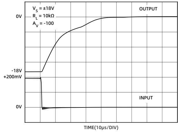
图 20 正过载恢复时间 (±18V)
