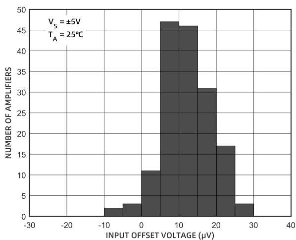
图 1 输入失调电压分布图 (±5V)
