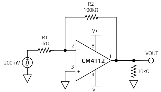
图 29 过载恢复时间的测试电路
