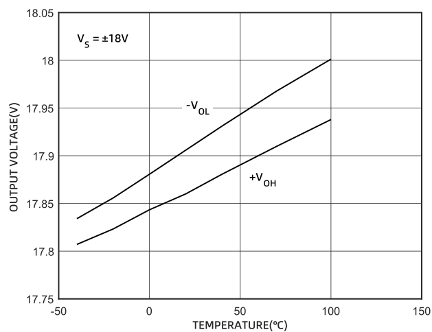
图 6 输出电压摆幅的温度特性 (±18V)
