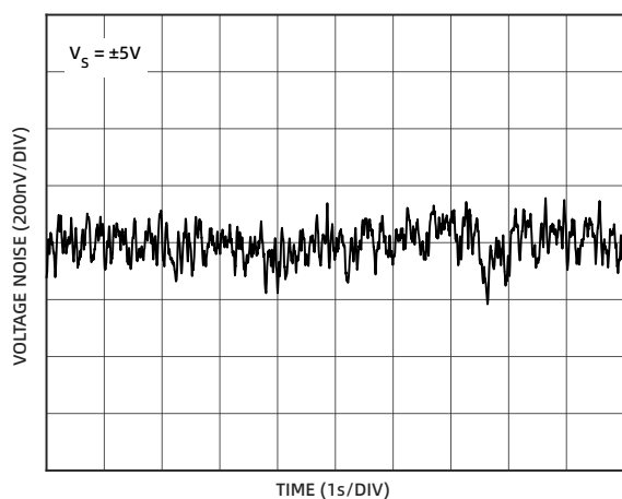
图 13 0.1Hz 至 10Hz 输入电压噪声 (±5V)
