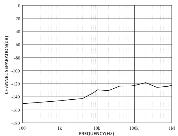
图 30 通道隔离度
