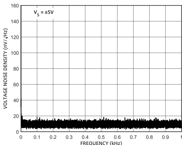
图 25 噪声频谱密度图 (±5V)
