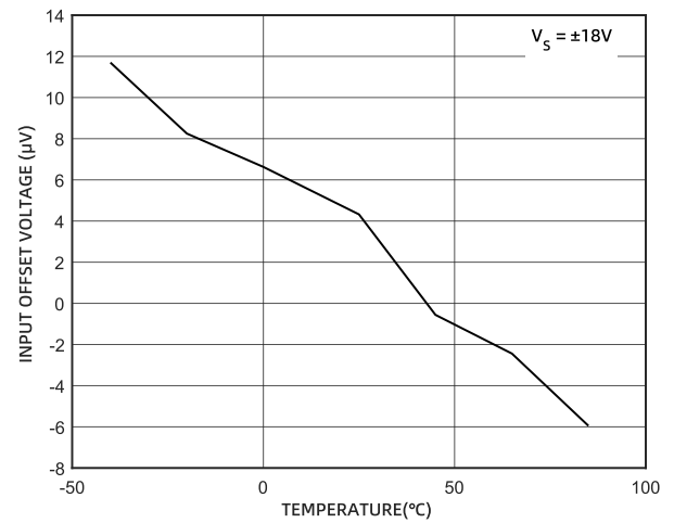
图 24 输入失调电压的温度特性 (±18V)
