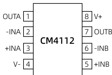
SOP8
