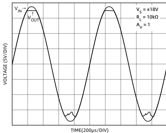
图 28 无反相 (±18V)
