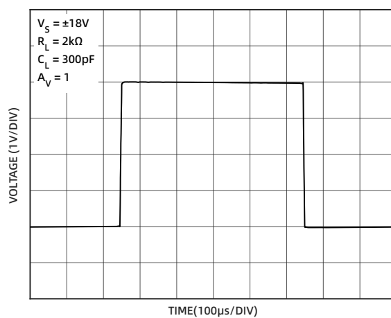
图 18 大信号瞬态响应 (±18V)
