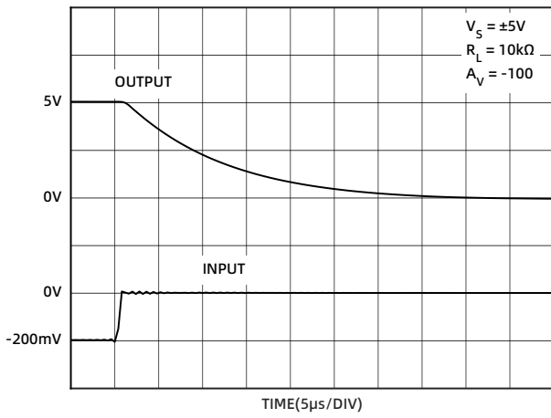
图 21 负过载恢复时间 (±5V)
