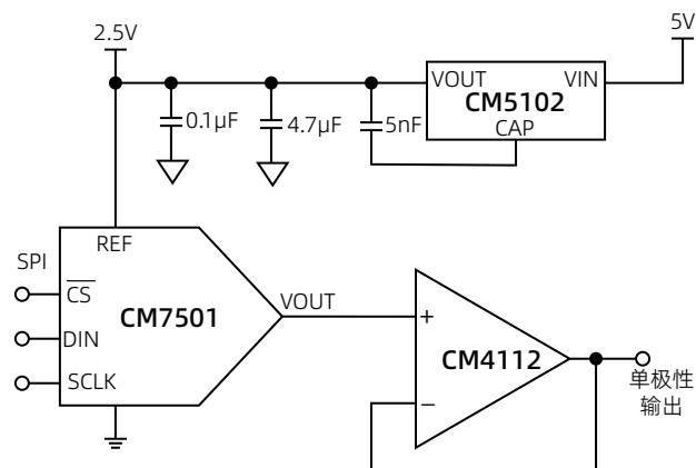
图 31 作为输出放大器
