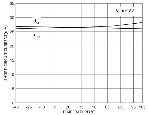
图 8 短路电流的温度特性 ( \pm 18V )
