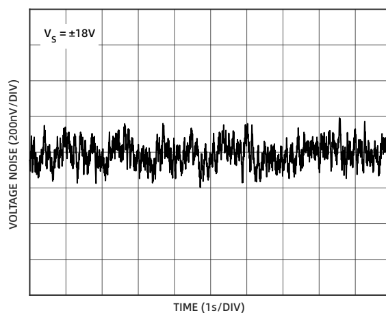
图 14 0.1Hz 至 10Hz 输入电压噪声 (±18V)
