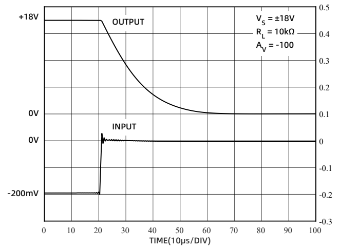
图 22 负过载恢复时间 (±18V)
