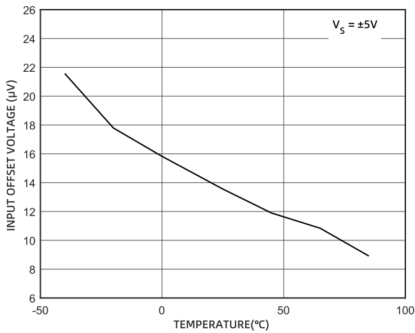
图 23 输入失调电压的温度特性 (±5V)
