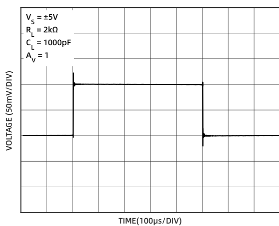
图 15 小信号瞬态响应 (±5V)
