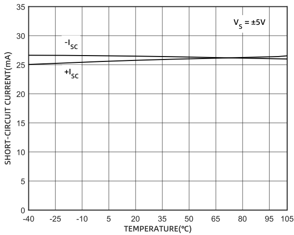
图 7 短路电流的温度特性 ( \pm 5V )
