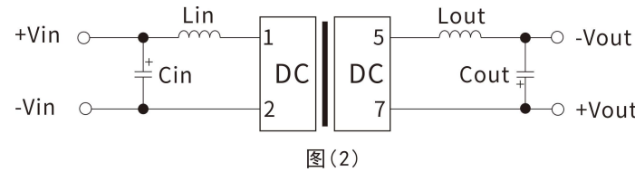
推荐 EMI 参考电路值详（表 2）
