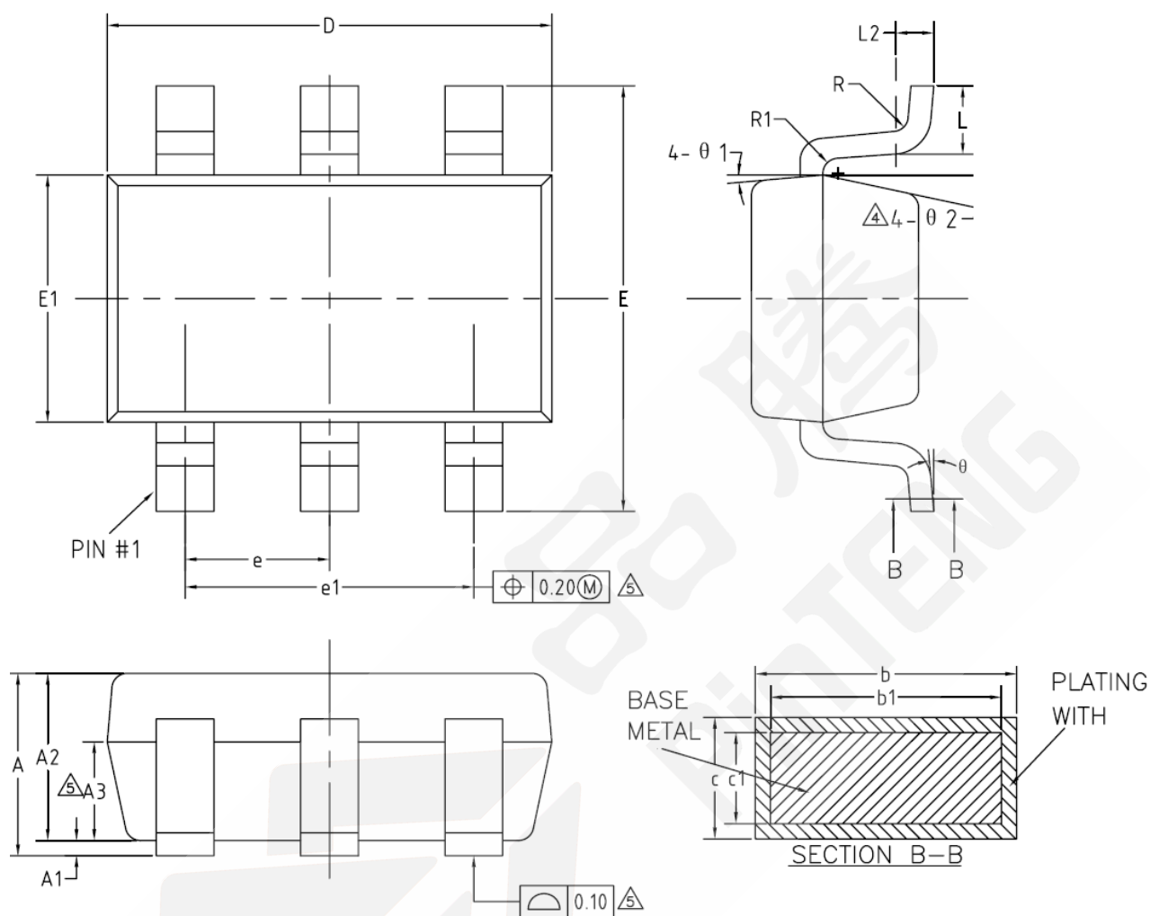
图 3 SOT23-6 封装图
