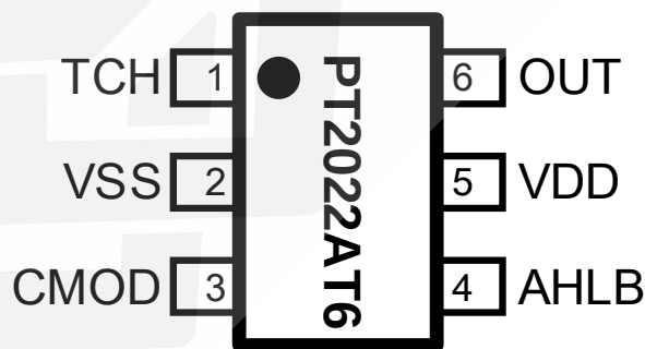
图 1 管脚示意
