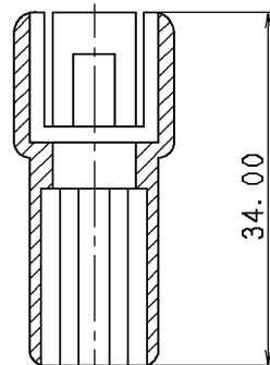
SEC. A-A
