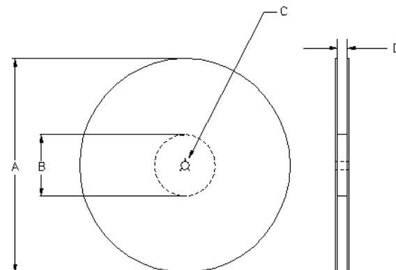
Reel Dimensions (1Kpcs) Table 3
