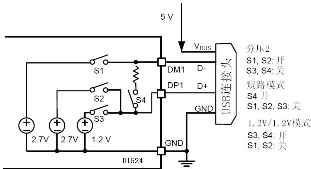
DCP 自动检测功能图表
