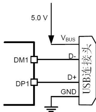
12W USB充电应用图
