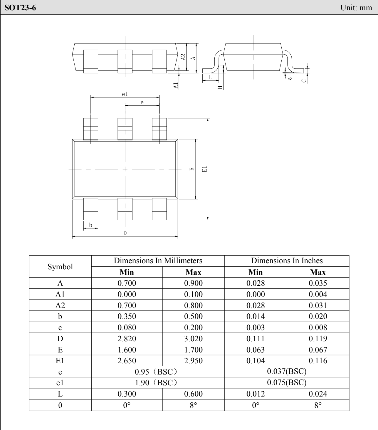
封装外形图:
