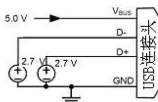
分压 3 DCP
