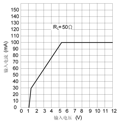
输入电流
