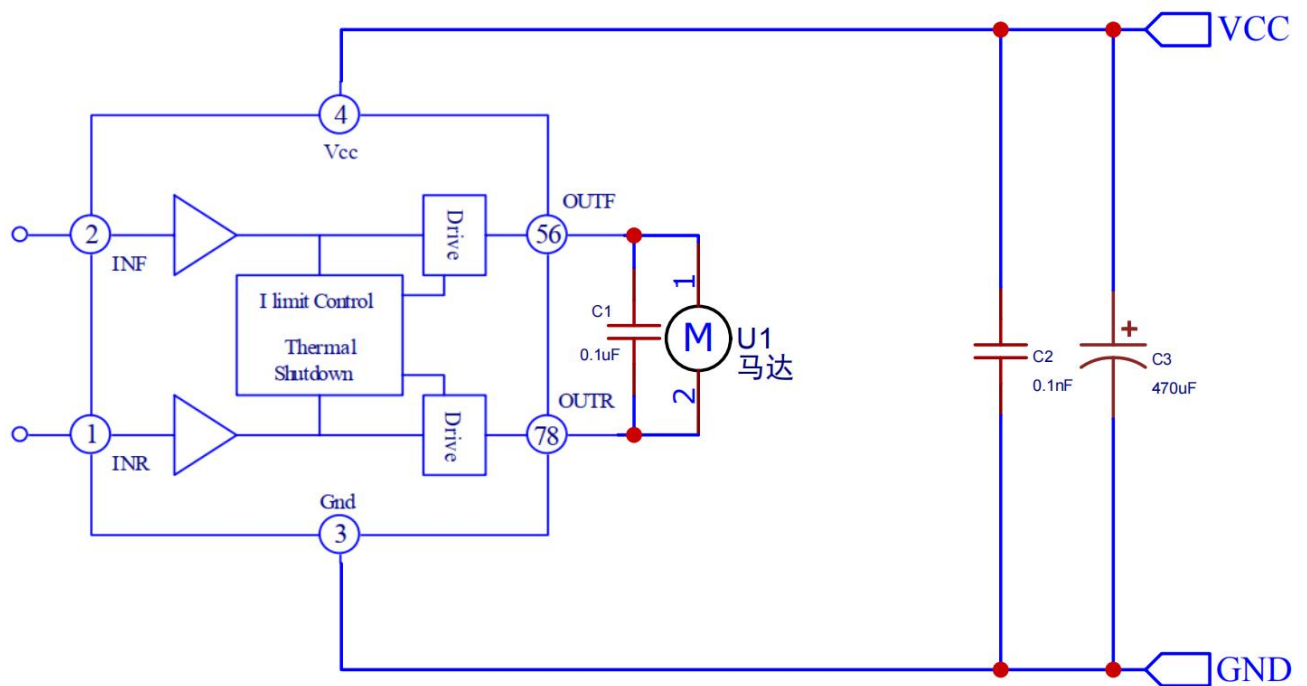
典型应用图:
