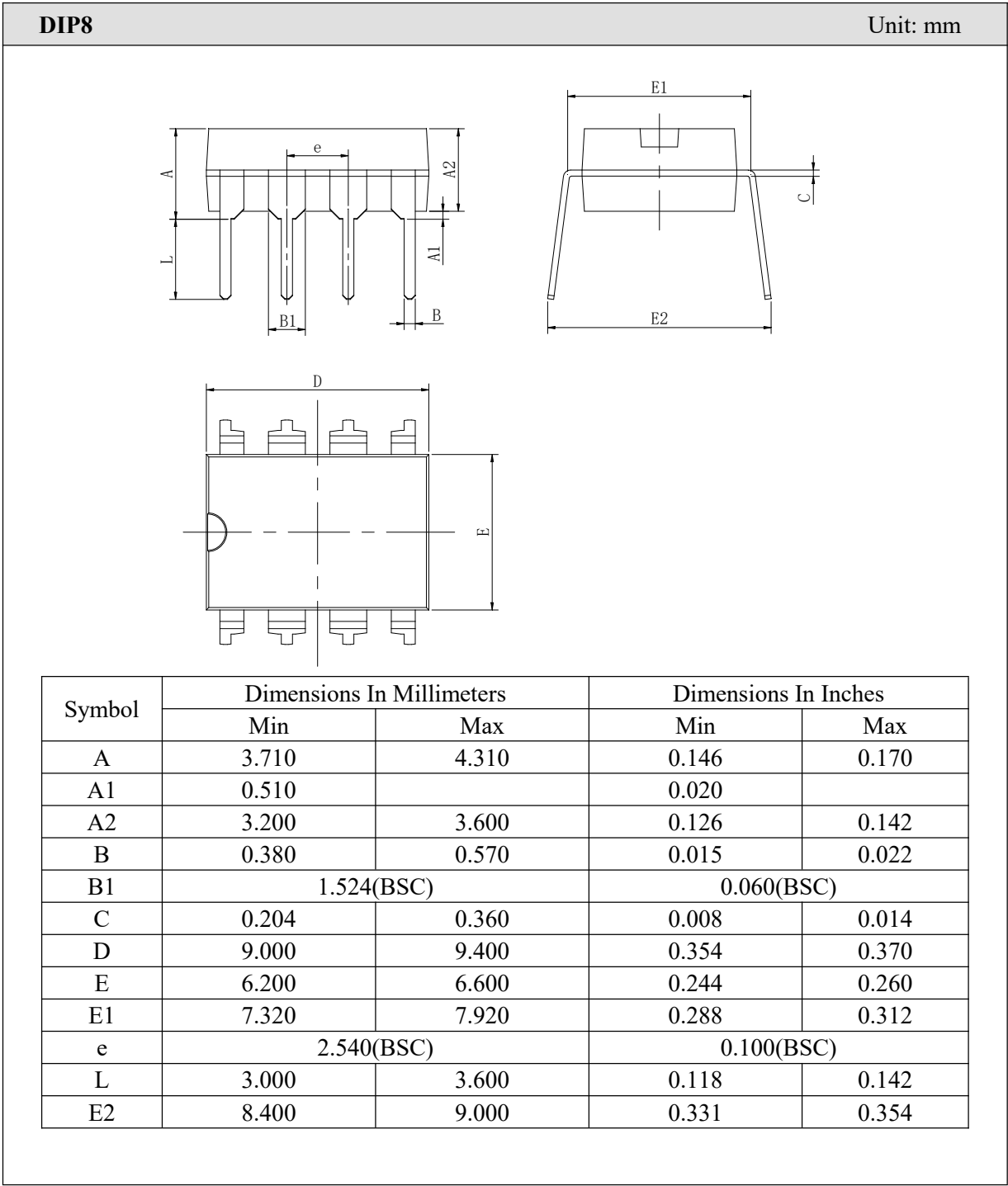
封装外形图:
