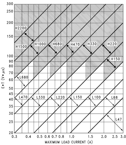
D2576HV-ADJ
