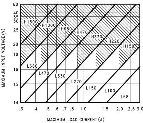
D2576HV-12
