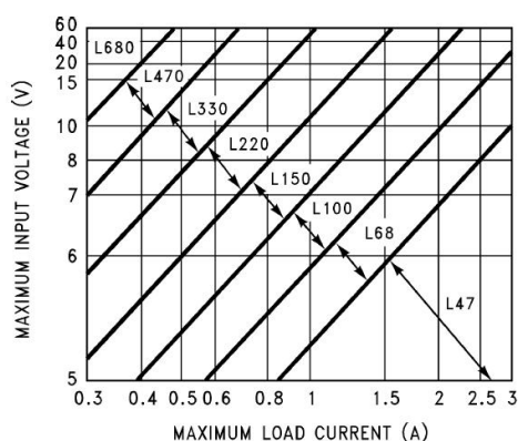
D2576HV-3.3
