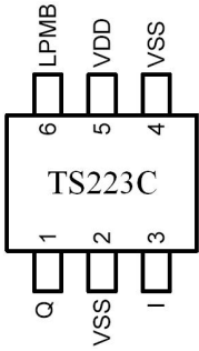
SOT23-6
