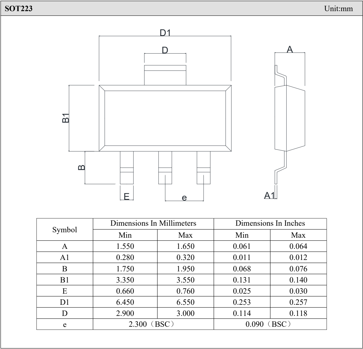
封装外形图：
