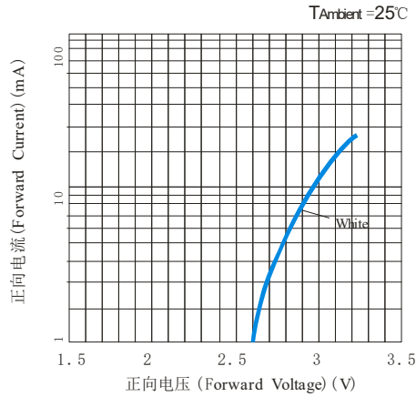
伏安特性
