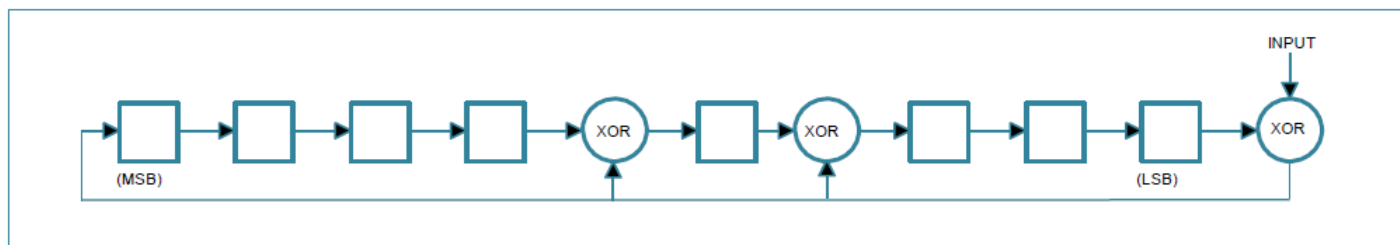
图 13 CRC 发生器
