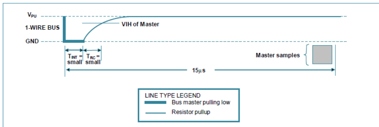
图 19 主机读 1 的详细时序
