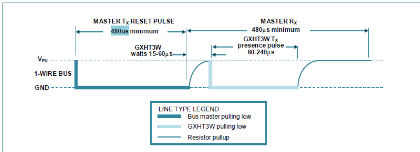
图 17 初始化时序
