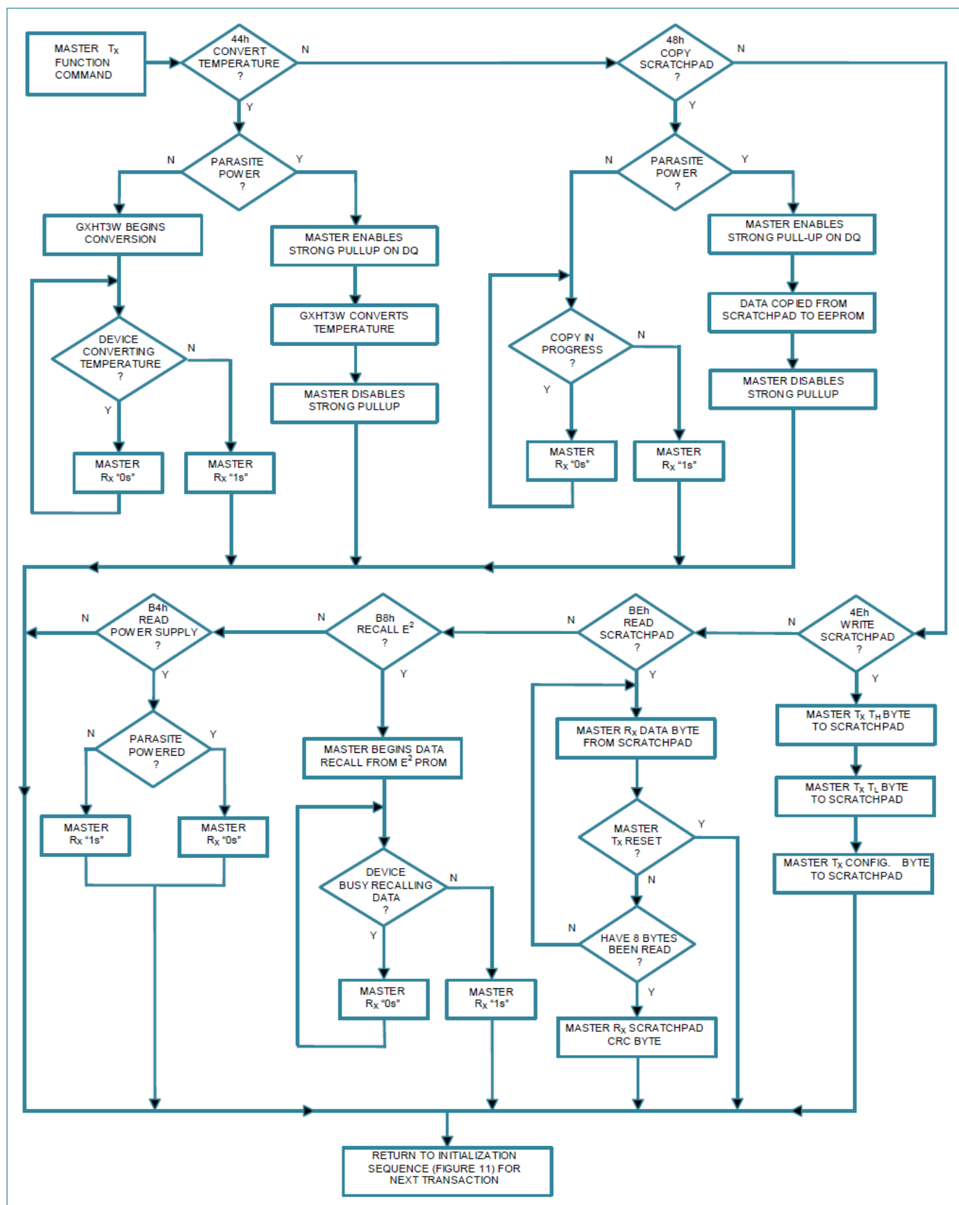
图 16 GXHT3W 功能指令流程图
