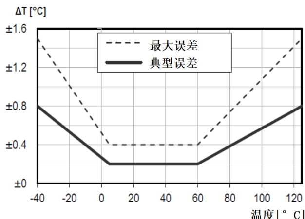
图 3 典型温度误差和最大温度误差
