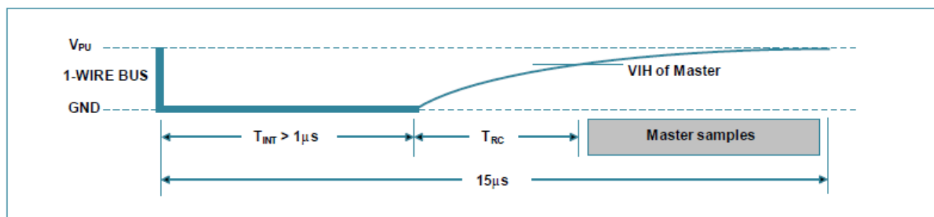
图 19 主机读 1 的详细时序
