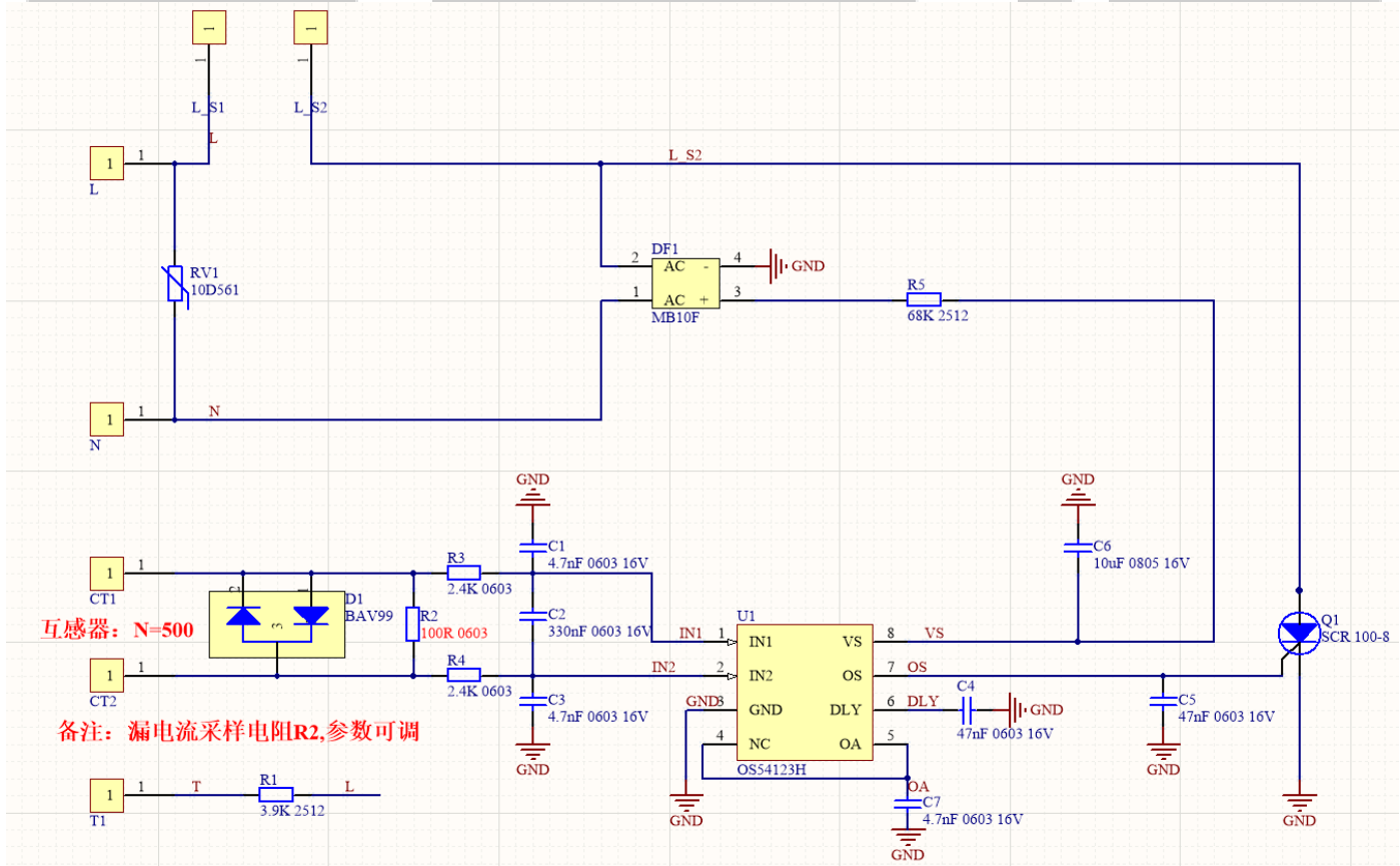
Figure 6. SS54123H 典型应用电路
