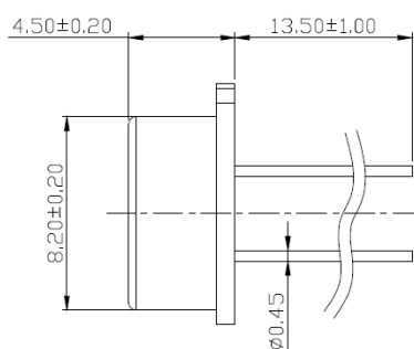
侧视图
