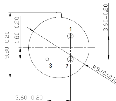
底视图
