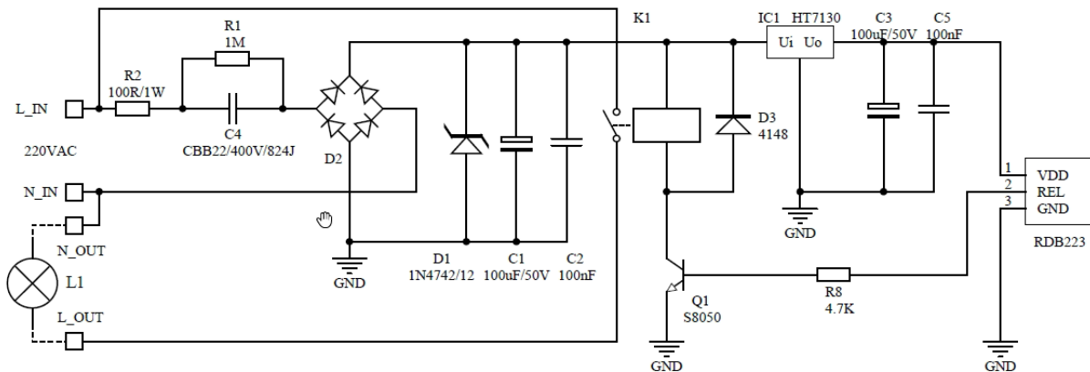
SYD-B223 数字热释电典型应用电路
