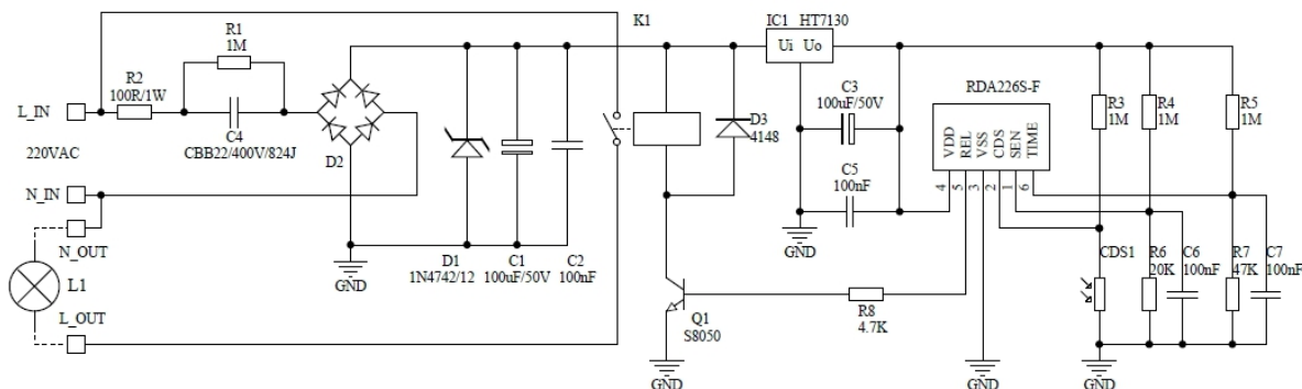
SYD-226S-F 数字热释电传感器典型参考电路
