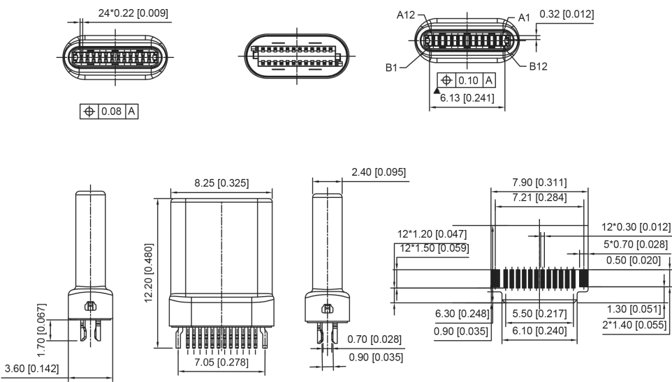
PLUG-USBC-241SMTV-4BS60
