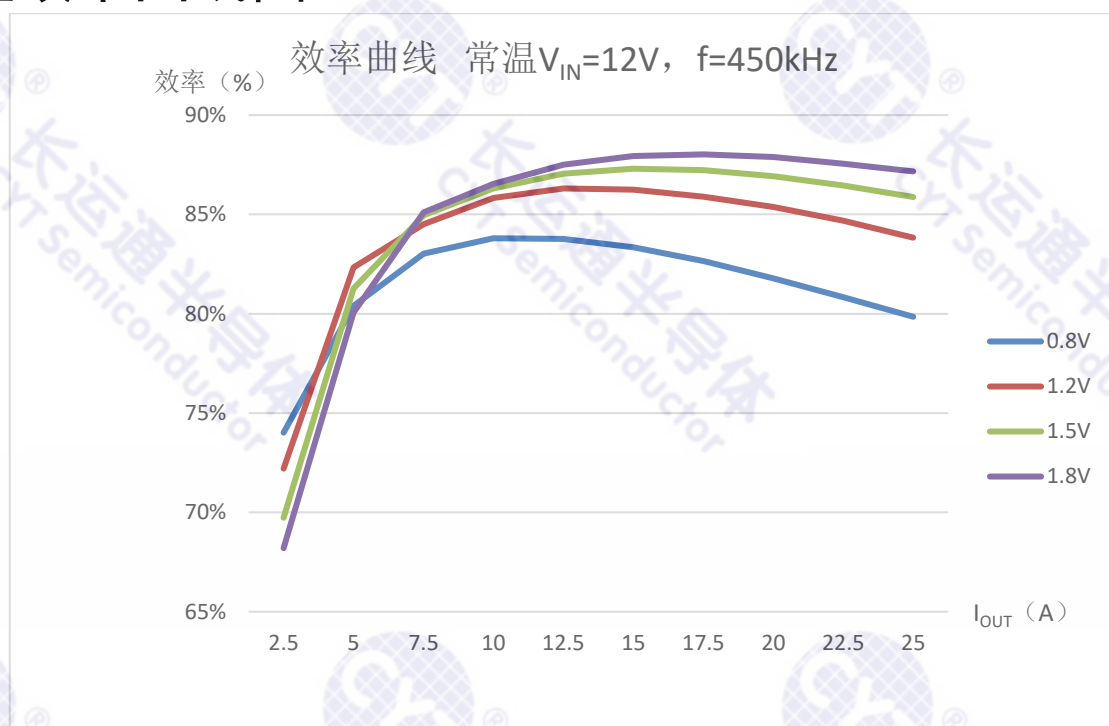
图 2 常温 V_{IN}=12V , f=450kHz 效率曲线图
