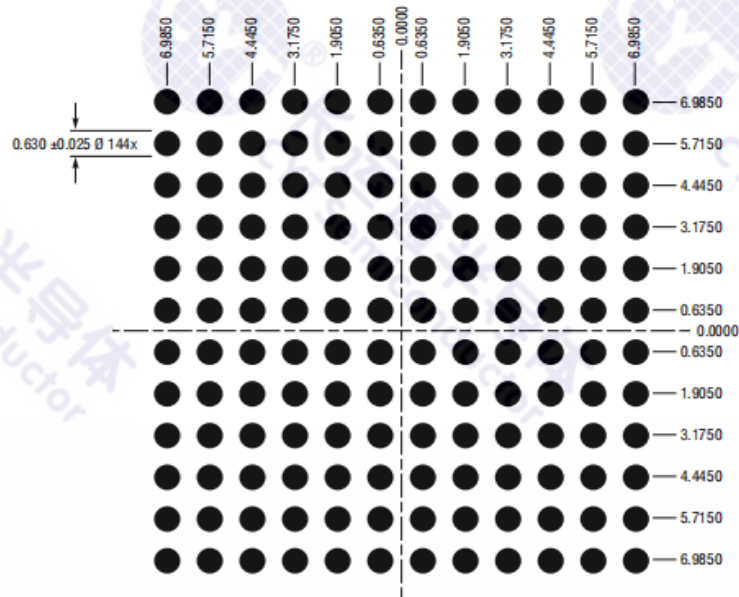
图7 脚位焊盘图 (BGA144)
