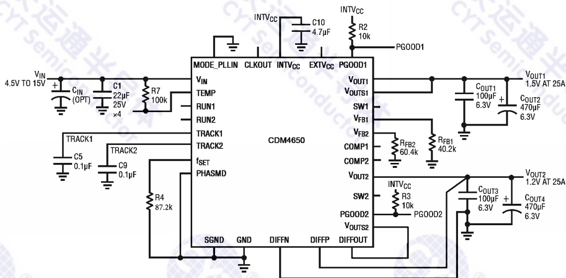
图6 V_{IN} : 4.5V~15V、双路1.5V和1.2V/25A输出
