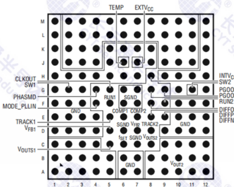
图1 脚位图 (16mm×16mm×5.01mm BGA144)
