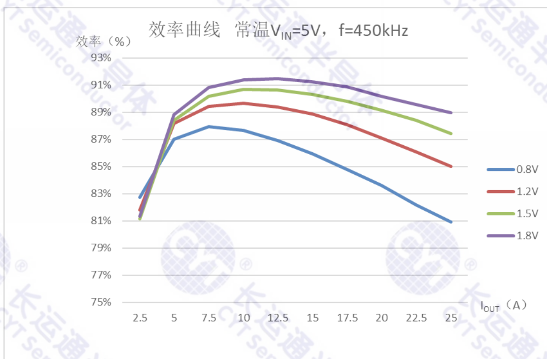
图3 常温 V_{IN}=5V , f=450kHz 效率曲线图
