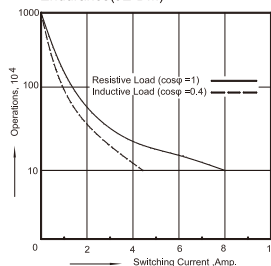
Endurance (JE-DM)
