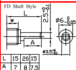
轴的类型:
