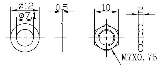
Washer 垫圈(可选项) Nut 螺母(可选项)
