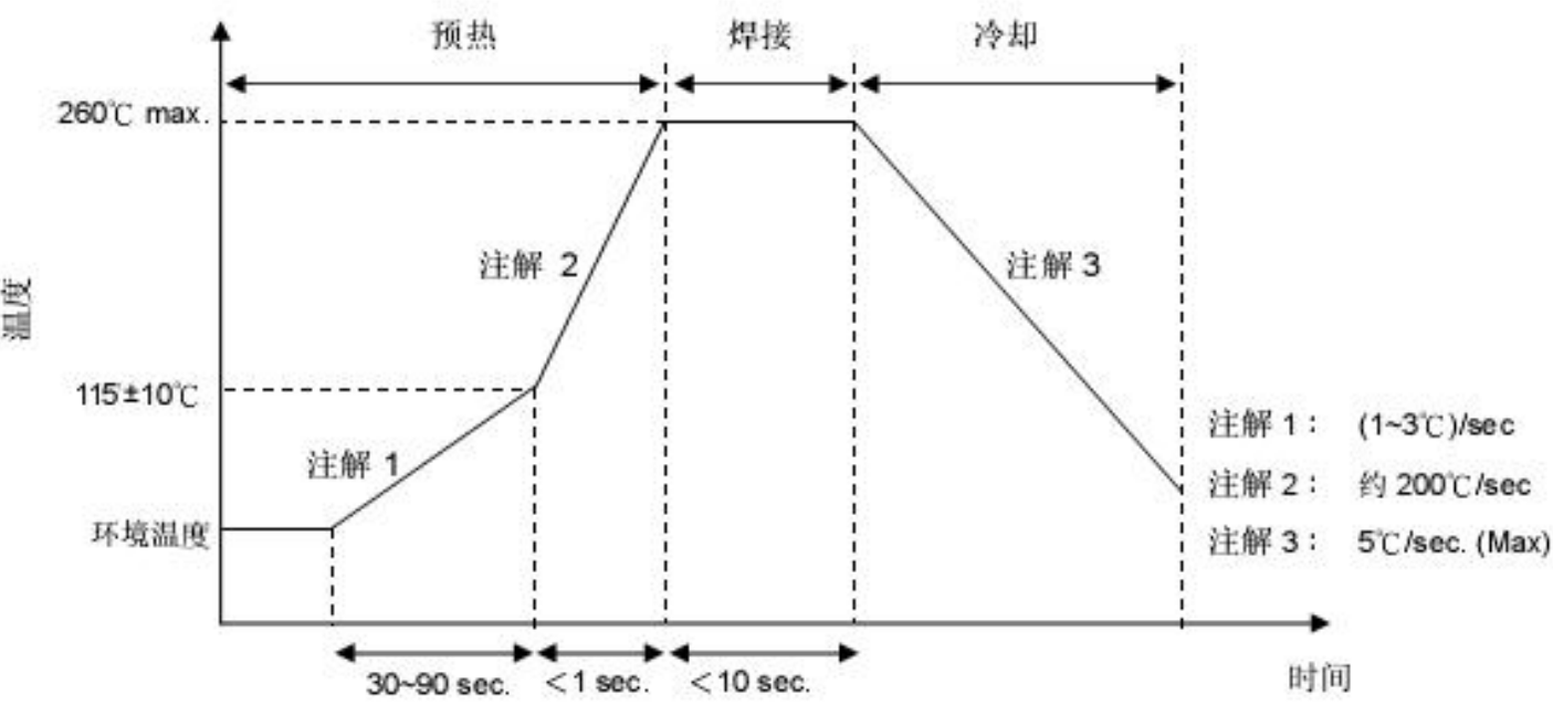
波峰焊曲线
