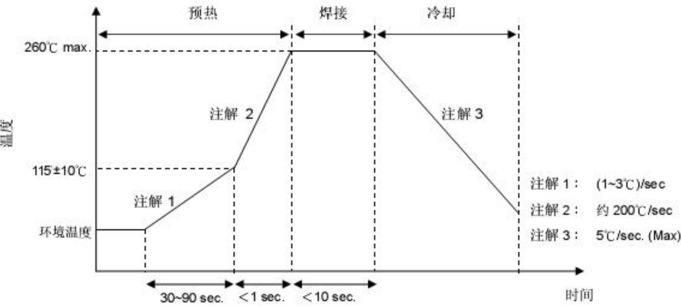
波峰焊曲线
