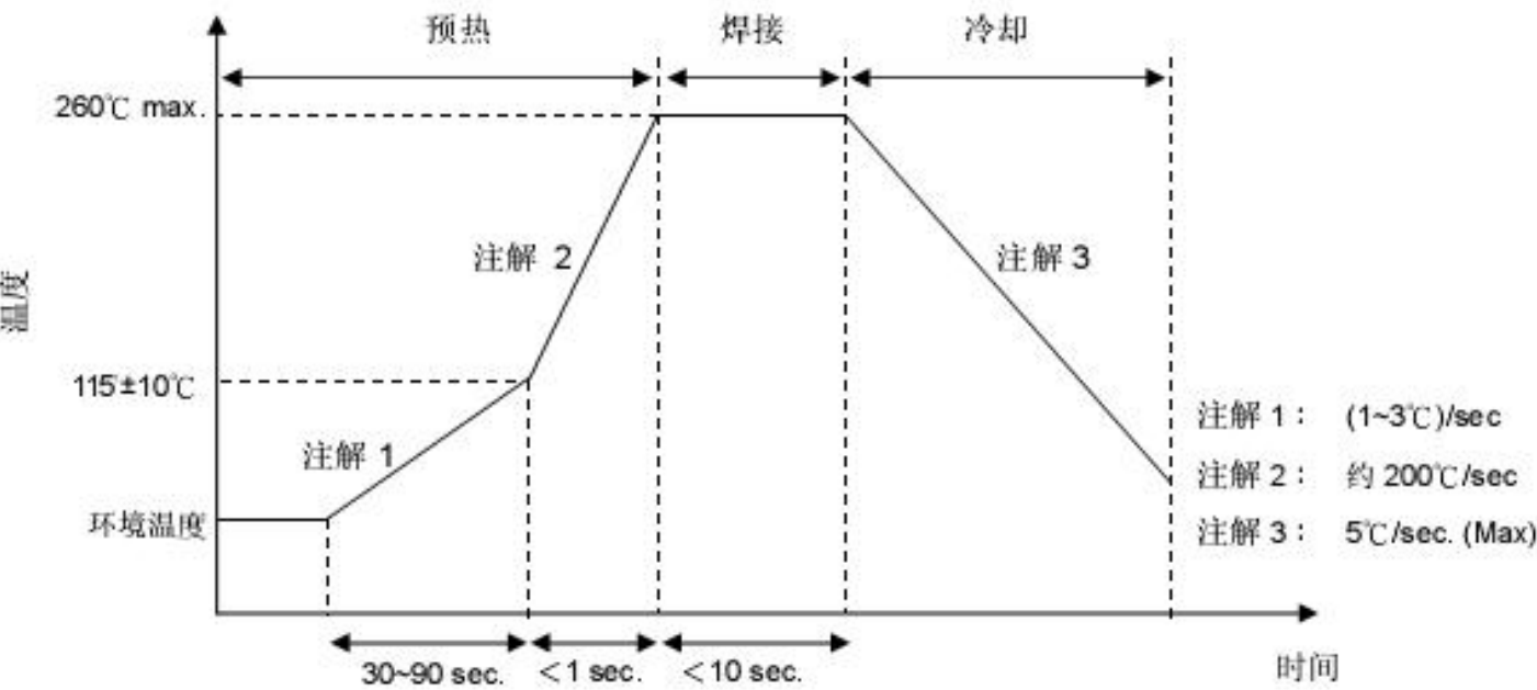
波峰焊曲线
