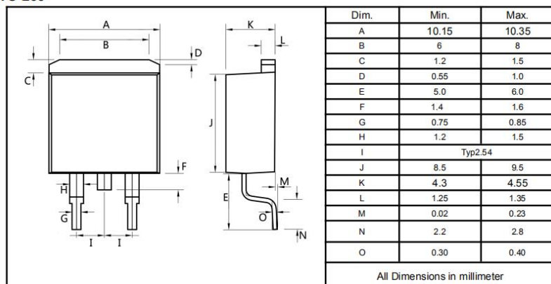
TO-263
