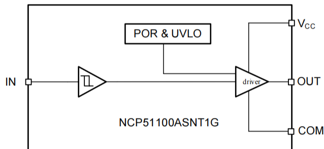
简化示意图
