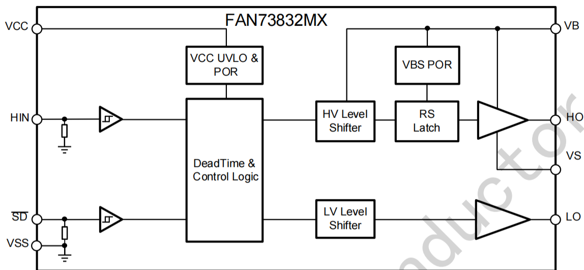
图 7-1 FAN73832的功能框图
