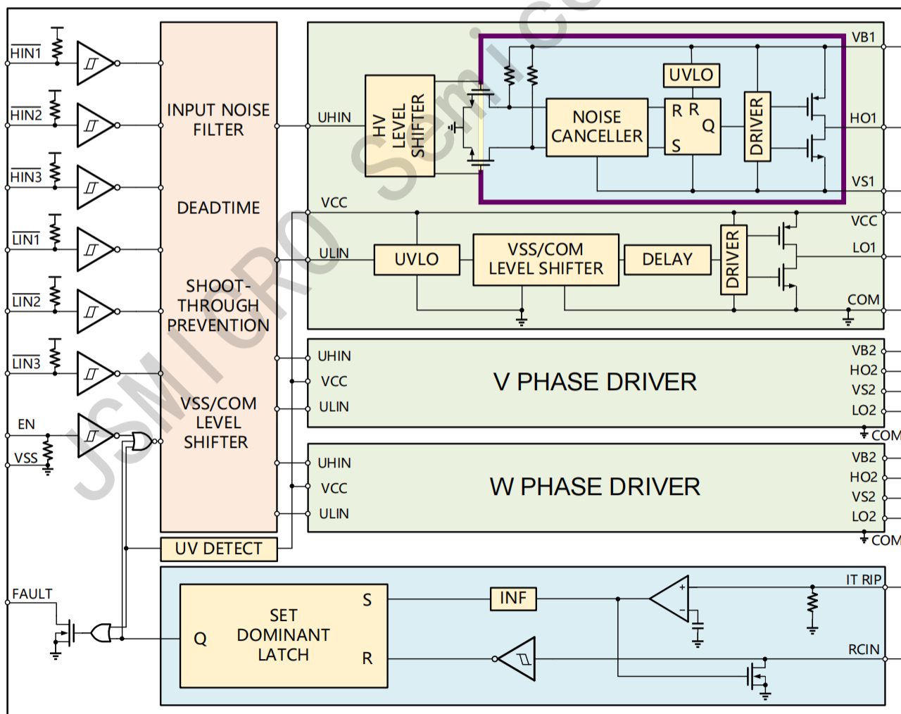
图7-1 FAN73892功能框图
