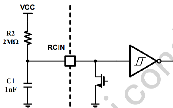
图 7-6 RCIN引脚框图
