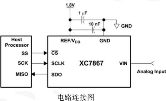
电路连接图
