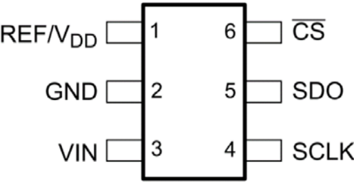
引脚图
