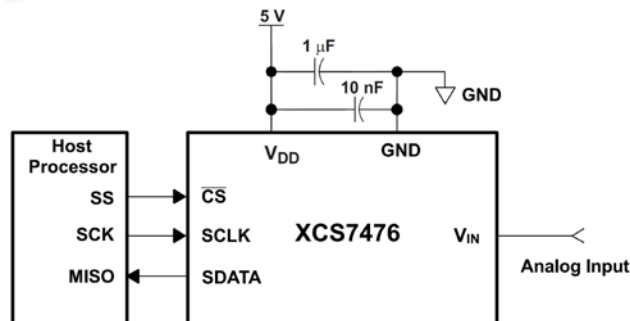
电路连接图
