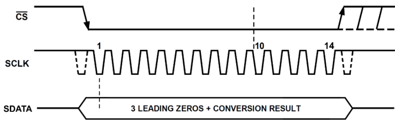
时序图
