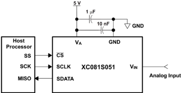
电路连接图
