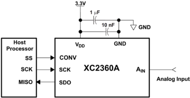
电路连接图
