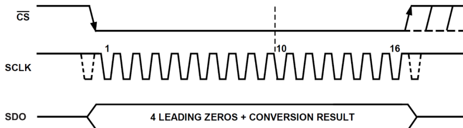
时序图
