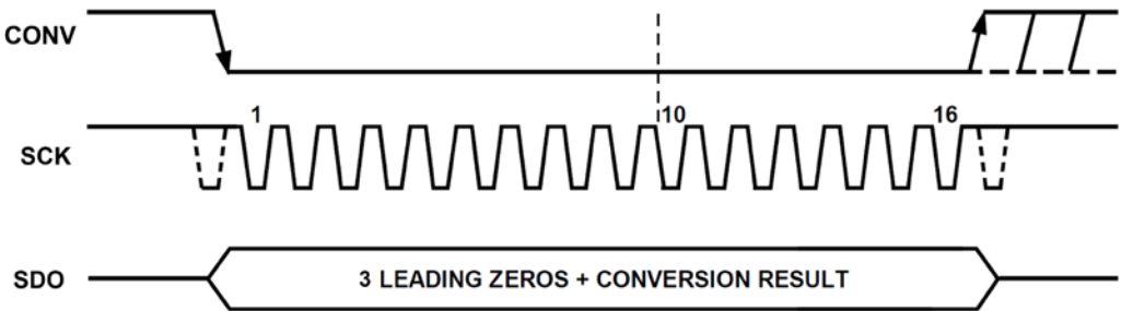
时序图
