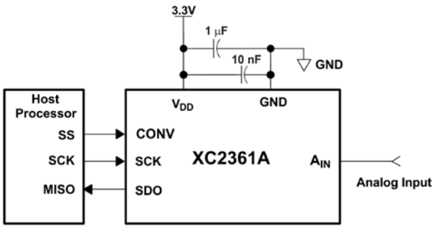
电路连接图
