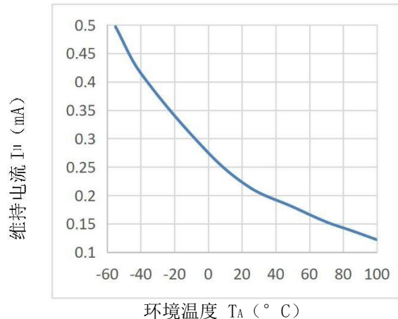
图5 维持电流 I_H vs 环境温度
