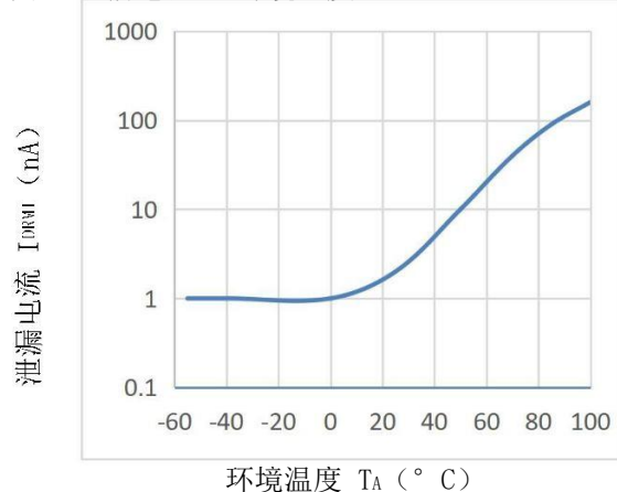
图6 泄漏电流 I_{DRM} vs 环境温度
