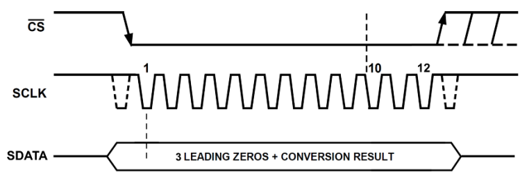
时序图
