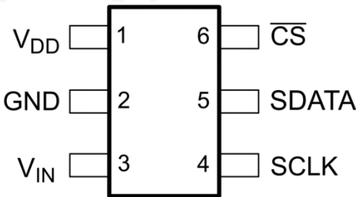
引脚图
