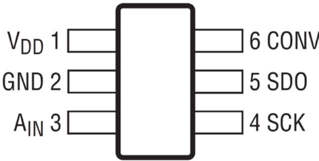
引脚图
